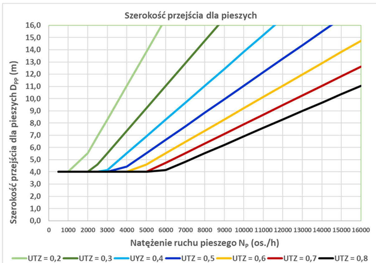
Rys. 10.2.1. Szerokości przejść dla pieszych z sygnalizacją świetlną D_{pp} w zależności od natężenia ruchu pieszego N_p i udziału światła zielonego dla pieszych w cyklu U_z
