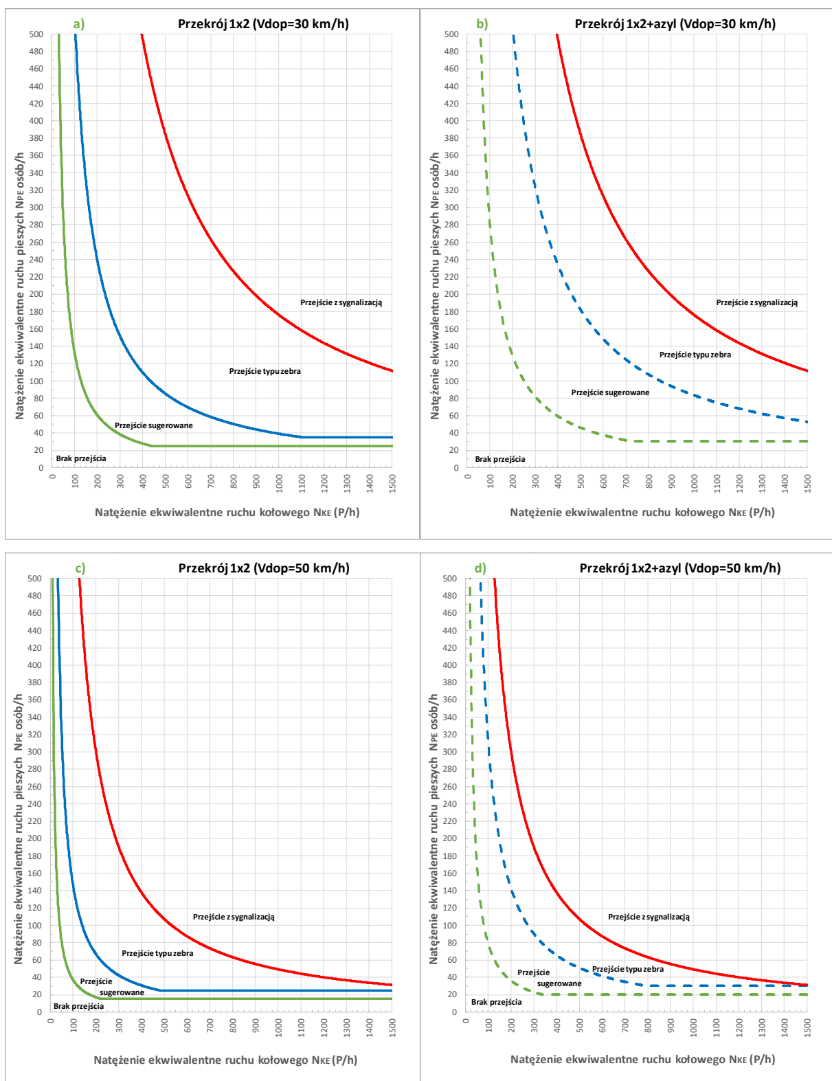
Rys. 8.4.3. Nomogram wyboru rodzaju infrastruktury punktowej dla pieszych przekraczających drogę o: a) V_{dop} = 30 \text{ km/h} bez wyspy azylu, b) V_{dop} = 30 \text{ km/h} z wyspą azylu, c) V_{dop} = 50 \text{ km/h} bez wyspy azylu, d) V_{dop} = 50 \text{ km/h} z wyspą azylu
